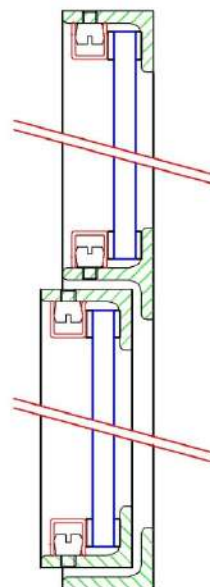
Coupe D-D
